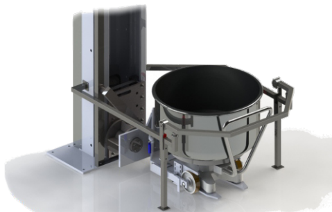
Sicherheitsbügel - Rohrgestell
